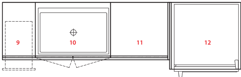
MẶT BẰNG TỦ BẾP DƯỚI 2
